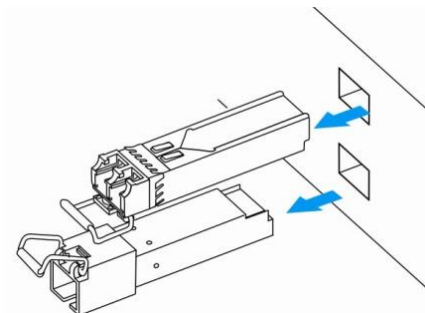
Рисунок 56 – Извлечение SFP-трансиверов
