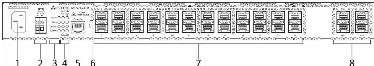
Рисунок 27 — Передняя панель MES2424FB
