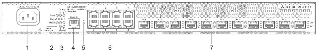
Рисунок 24 – Передняя панель MES2411X
