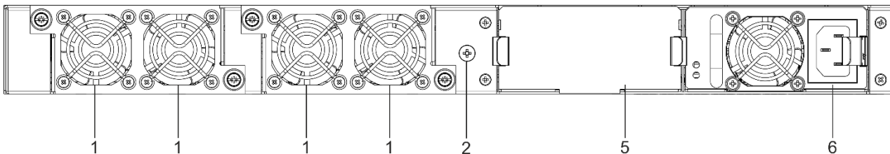
Рисунок 36 – Задняя панель MES2420-48P
