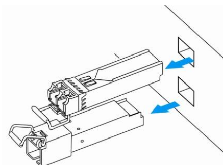
Рисунок 55 – Извлечение SFP-трансиверов
