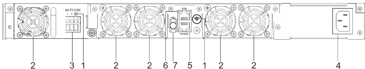
Рисунок 23 – Задняя панель MES5400-48
