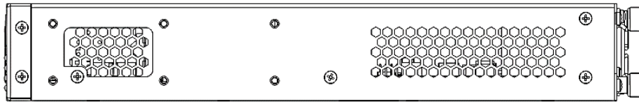
Рисунок 33 – Правая боковая панель MES5316A, MES5324A, MES5332A
