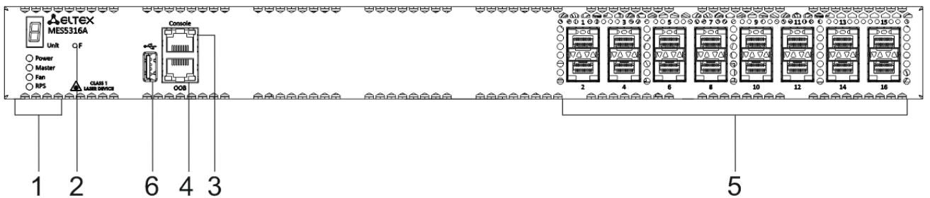
Рисунок 8 – Передняя панель MES5316A
