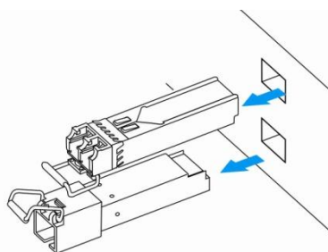
Рисунок 28 – Извлечение SFP-трансиверов
