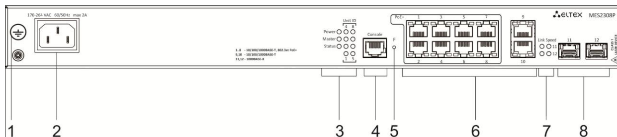
Рисунок 8 – MES2308P, передняя панель
