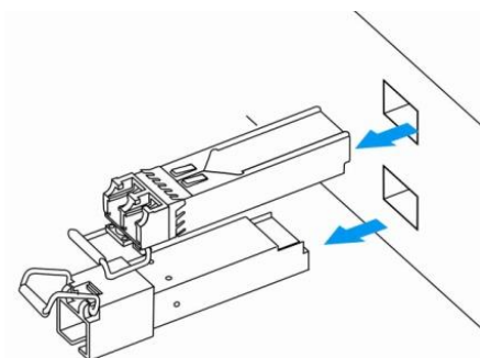
Рисунок 55 – Извлечение SFP-трансиверов
