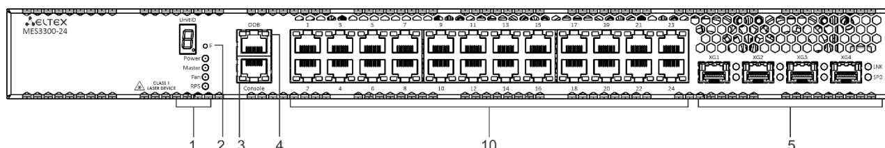
Рисунок 4 – Передняя панель MES3300-24
