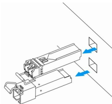
Рисунок 28 – Извлечение SFP-трансиверов
