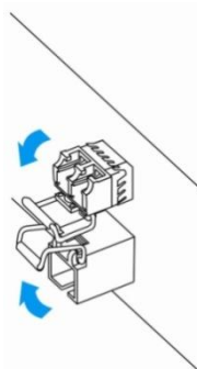
Рисунок 27 – Открытие защелки SFP-трансиверов
