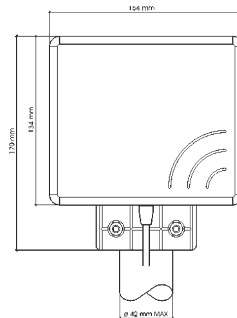
Установка на мачту
