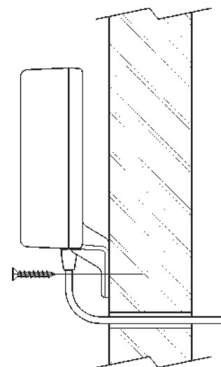
Установка на стену (винты в комплект не входят)
