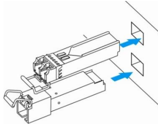
Рисунок 47 — Установка SFP-трансиверов
