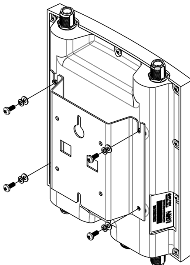
Рисунок 11 – Крепление кронштейна
