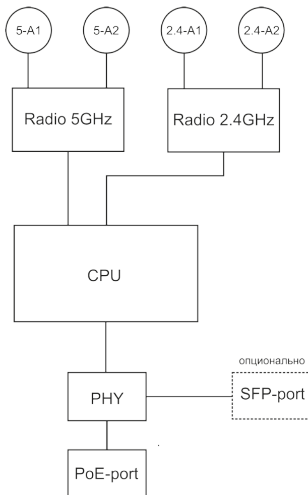
Рисунок 2 – Структурная схема WOP-2ас
