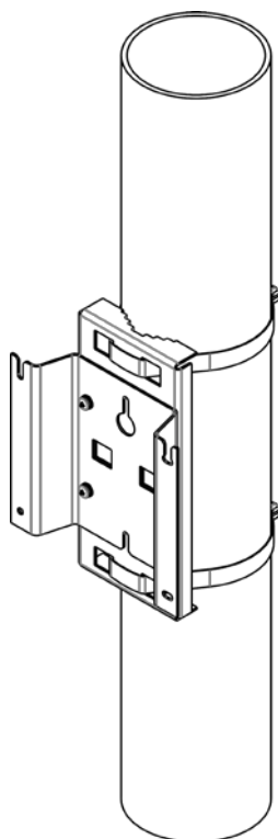
Рисунок 8 – Крепление кронштейна на трубостойку
