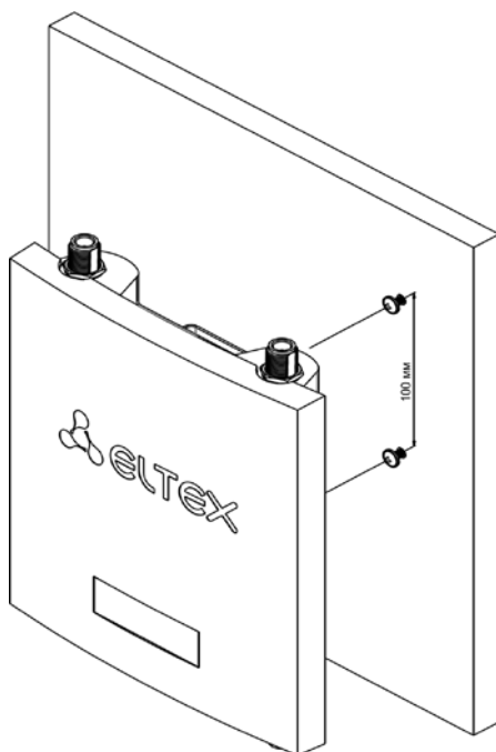
Рисунок 12 – Крепление устройства на стене
