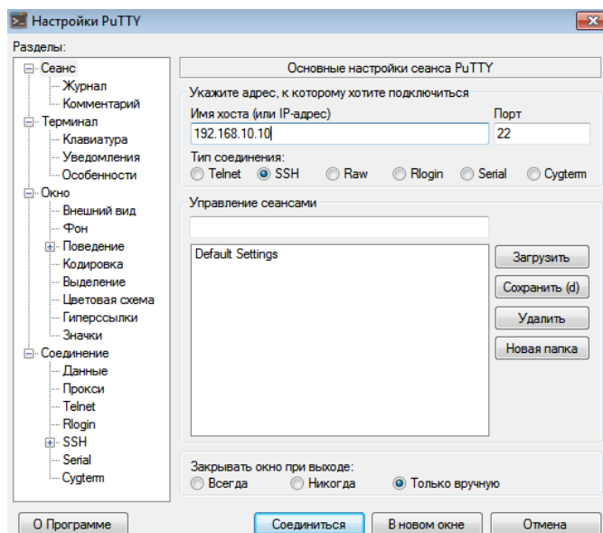
Рисунок 2 – Запуск SSH-клиента
