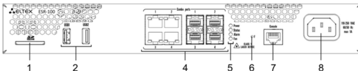
Рисунок 36 – Передняя панель ESR-100
